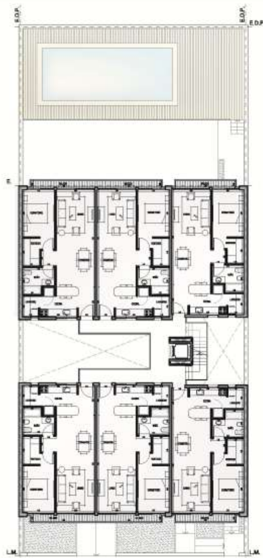
PLANTA 2º y 3º PISO
